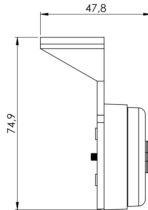
Front position lamp HOR 123, with hanger Lampa pozycyjna przednia HOR 123, z wieszakiem
